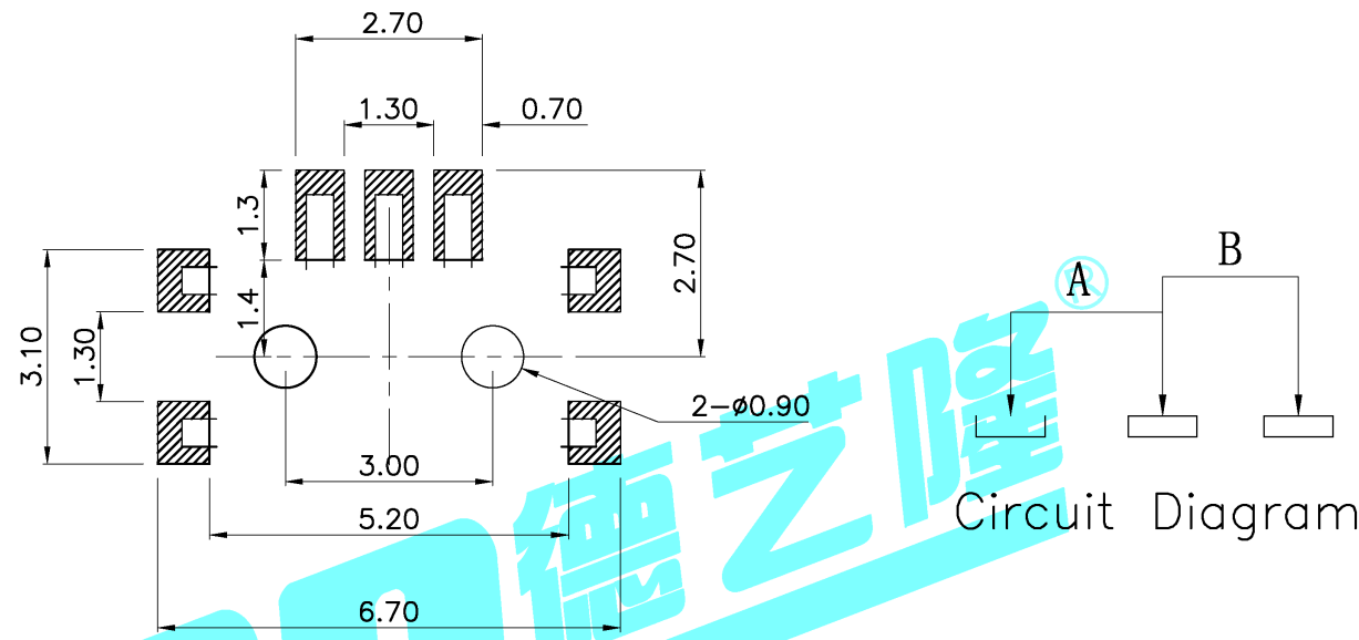
PCB Layout(Pattern side)
