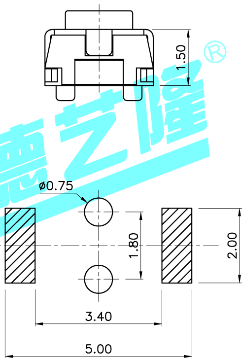
PCB Layout(Pattern Side)
